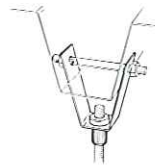
LTV - voor dakprofielen
